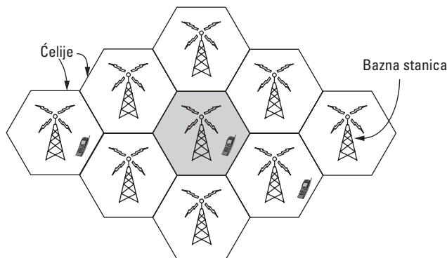
Slika 1-30. Podela mreža mobilne telefonije na ćelije.
