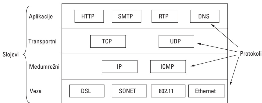
Slika 1-22. Model TCP/IP i neki protokoli koje ćemo proučavati.
