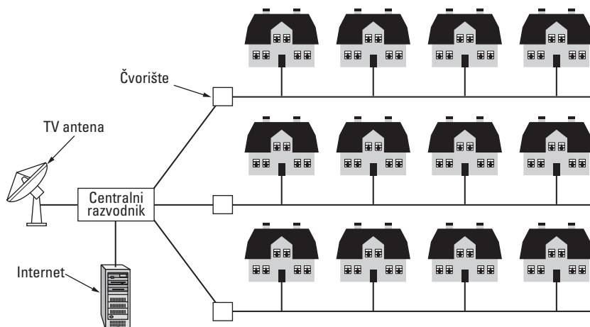
Slika 1-9. Gradska mreža zasnovana na sistemu kablovske televizije.
