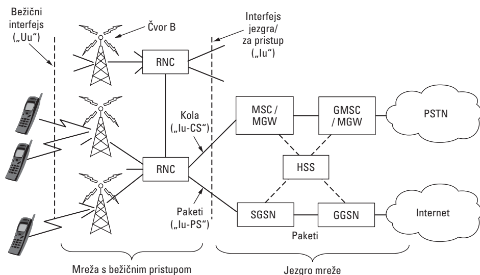
Slika 1-31. Arhitektura 3G mobilne telefonske UMTS mreže.
