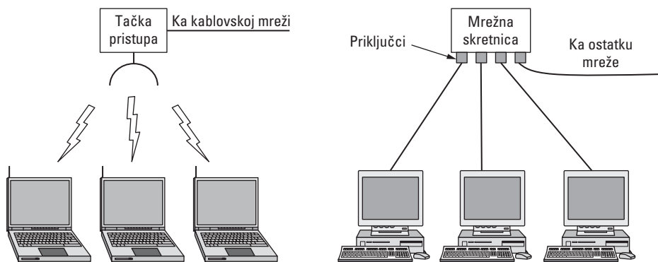
Slika 1-8. Bežična i ožičena lokalna mreža. (a) 802.11 (b) Komutirani Ethernet.
