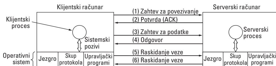
Slika 1-18. Razmena paketa tokom jednostavne komunikacije između klijenta i servera pomoću datagrama s potvrdom o prijemu.
