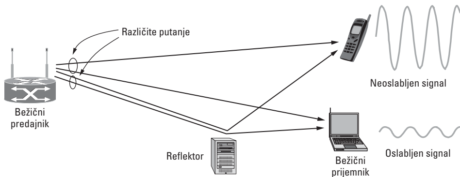
Slika 1-34. Slabljenje zbog različitih putanja.
