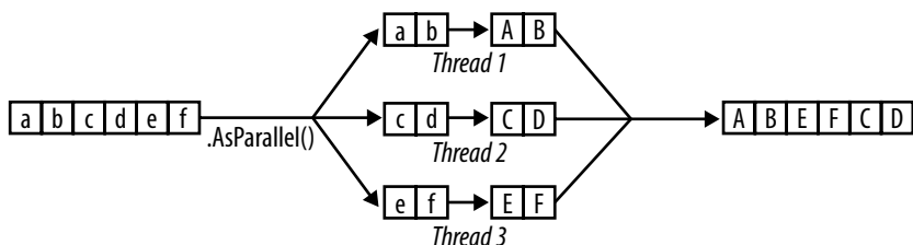
Slika 23-2. PLINQ-ov model izvršavanja.
