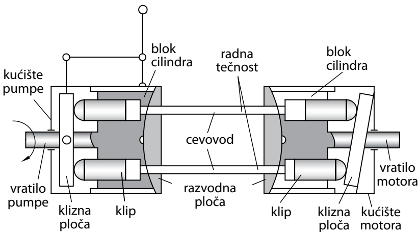
Slika 1.6 Pojednostavljen prikaz hidrauličnog sistema sa zapreminskim upravljanjem.
