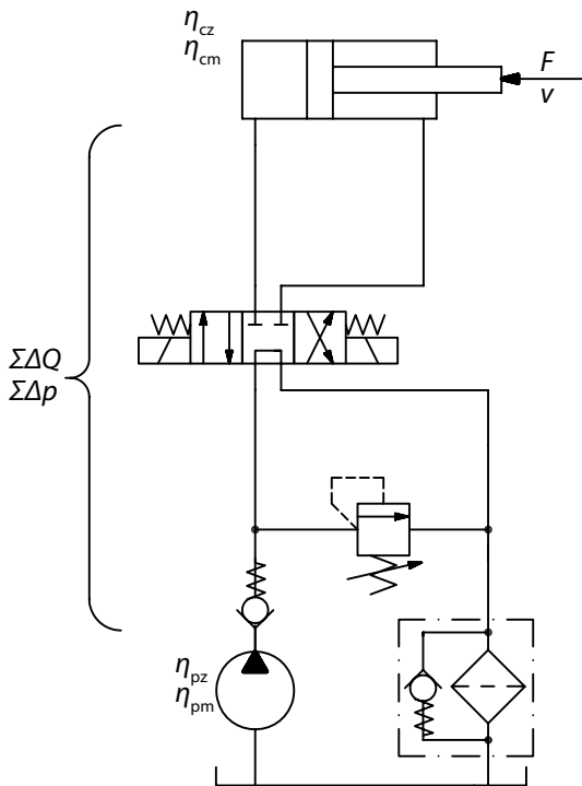
Slika 1.10 Funkcionalna šema hidrauličnog sistema.
