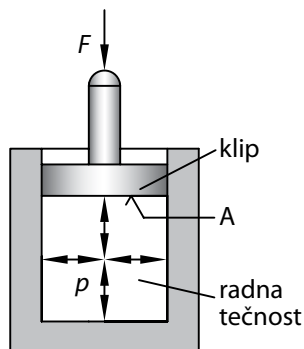
Slika 1.1 Stvaranje pritiska u zatvorenom cilindru.
