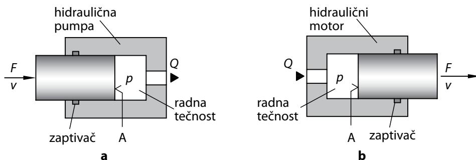
Slika 1.8 Elementarna hidraulična pumpa (a) i hidraulični motor (b).
