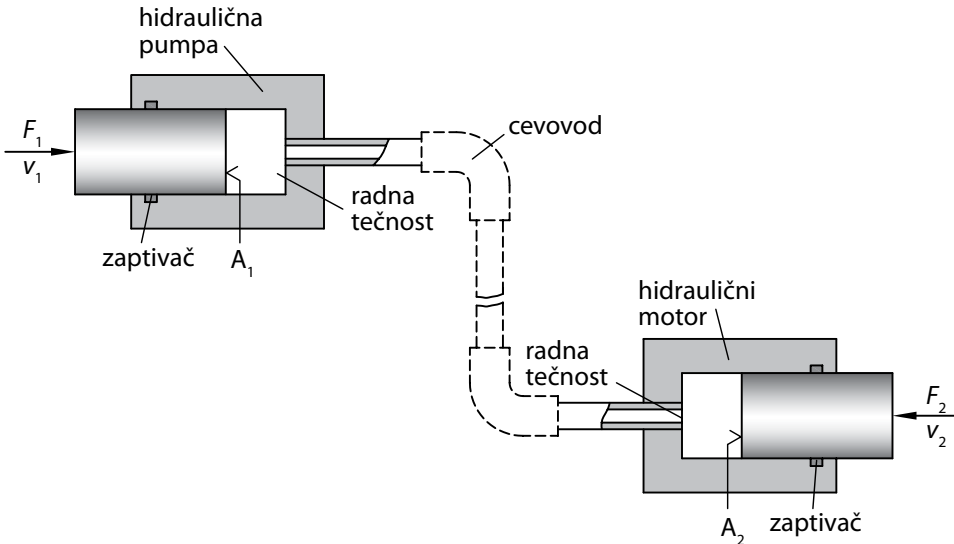
Slika 1.3 Idealan hidraulični prenosnik.
