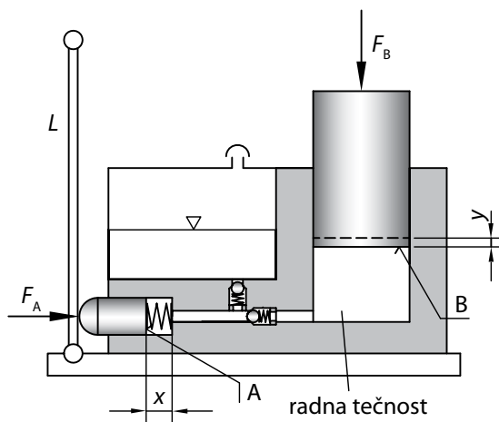
Slika 1.2 Hidraulični sistem – hidraulična dizalica.
