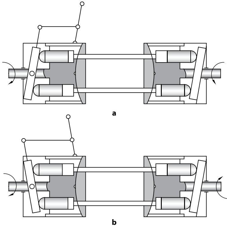
Slika 1.7 Upravljanje smerom i brzinom rotacije vratila hidromotora (a i b).
