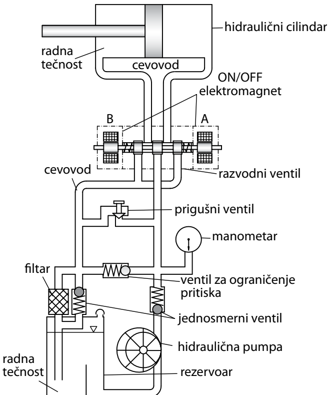
Slika 1.4 Pojednostavljen prikaz hidrauličnog sistema s prigušnim upravljanjem.
