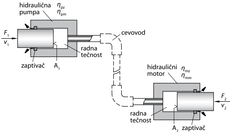
Slika 1.9 Šematski prikaz realnog hidrauličnog prenosnika.
