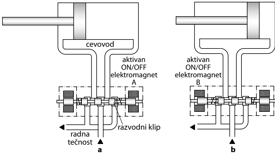
Slika 1.5 Izvlačenje klipnjače hidrauličnog cilindra (a) i uvlačenje klipnjače (b).
